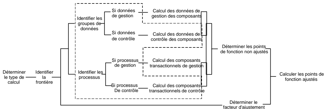
Figure 2 – Diagramme de la procédure de calcul des PFCs
