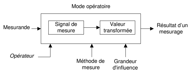
Figure 9 Processus de mesure – Topologie détaillée des sous-concepts
