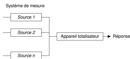
Figure 14 Modèle d'un appareil de mesure totalisateur
