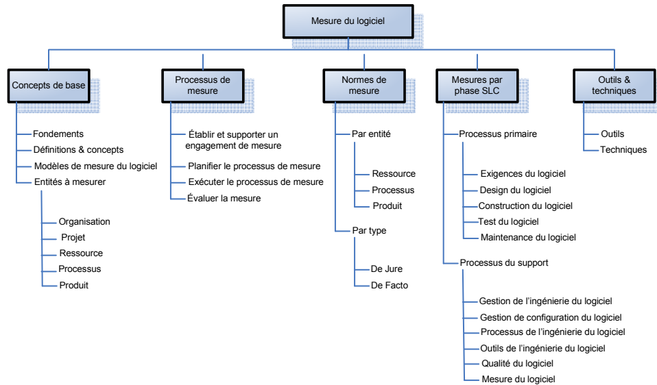
Figure 43 Taxonomie pour KA de mesure de logiciels dans SWEBOK [27]
