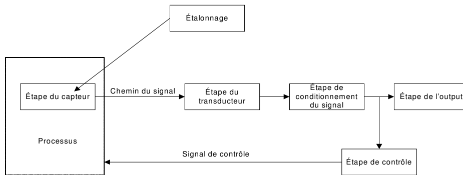
Figure 27 Composants d'un système de mesure général [43]
