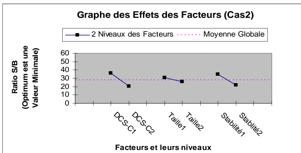
Figure 8.4 Graphe des effets des facteurs (Cas 2).
