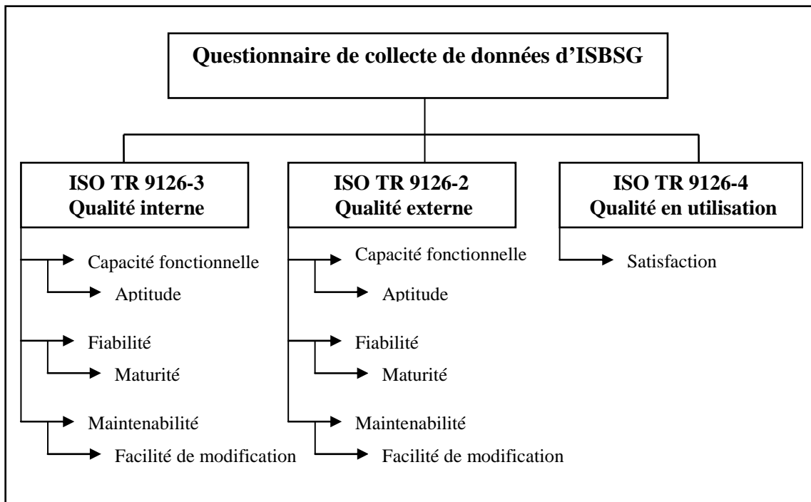
Figure 6.1 Récapitulatif de l'analyse du questionnaire d'ISBSG selon ISO TR 9126-2 à 4.
