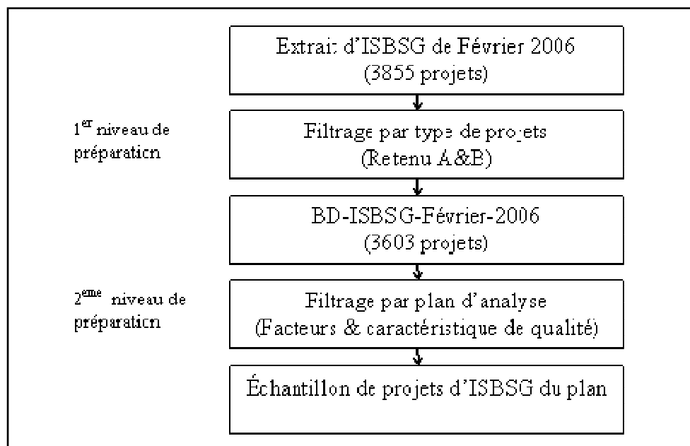
Figure 7.1 Étapes de préparation des données d'ISBSG.
